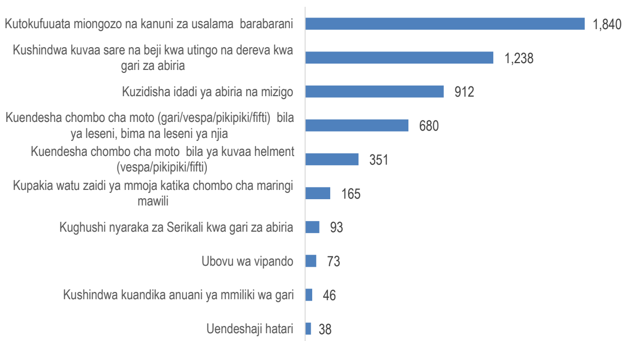
Kielelezo 2.1: Idadi na Aina ya Makosa ya Barabarani, Julai 2024
